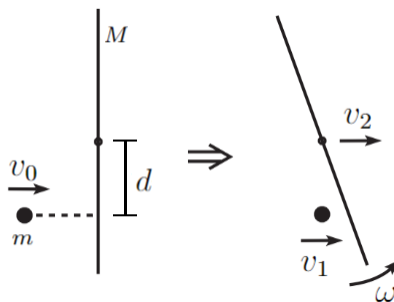
Figura 1: Schematizzazione dell'urto tra una palla e un'asta non vincolata.
