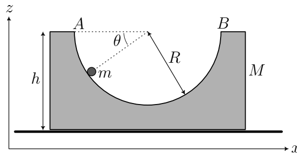
Figura 8: Disegno schematico della prima configurazione del Problema 6.8.
