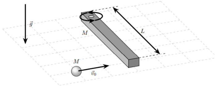
Figura 7: Schematizzazione dell'urto tra la palla e l'asta non omogenea.
