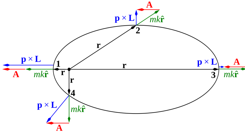
Figura 3: Orientazione del vettore di Lenz, calcolato in quattro punti diversi dell'orbita.
